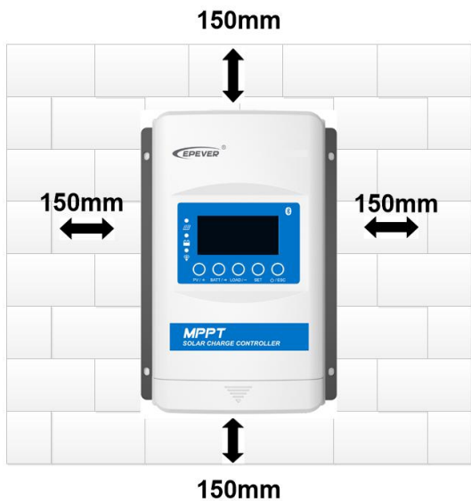
图2-1安装示意图
