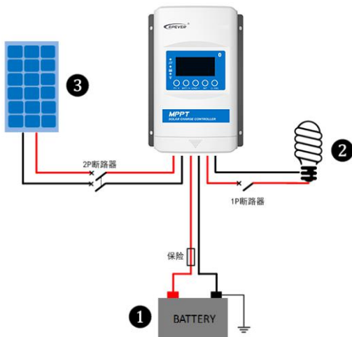
图2-2接线示意图
